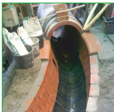
zdění kanalizačních objektů
